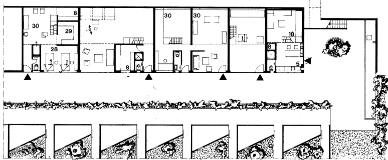
STRASSENGESCHOSS
