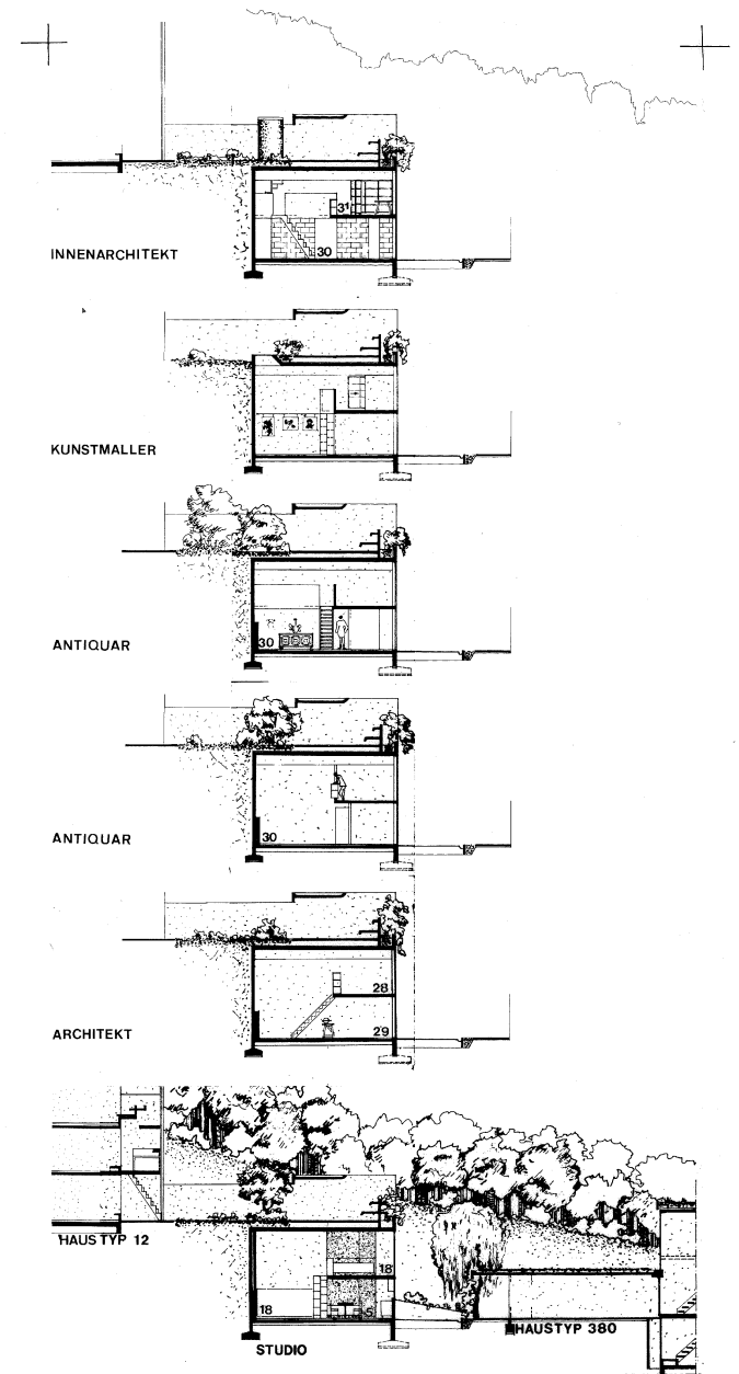
LÄNGSSCHNITT
