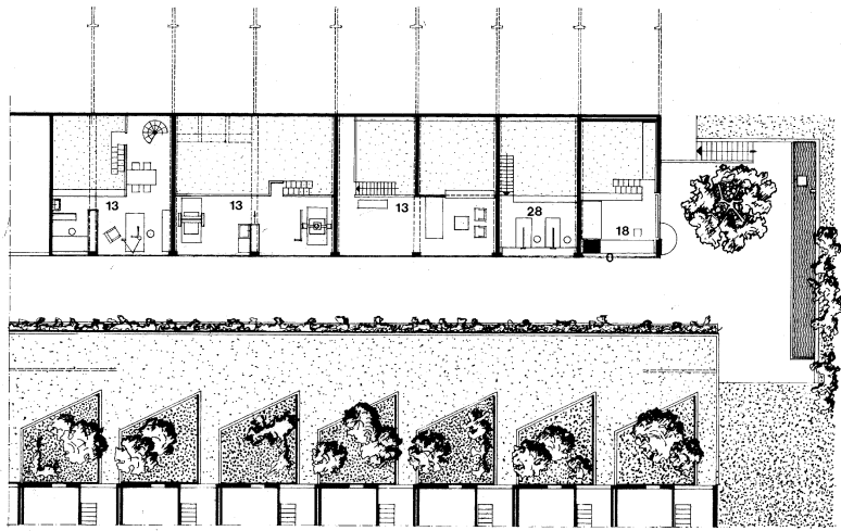
OBERGESCHOSS
