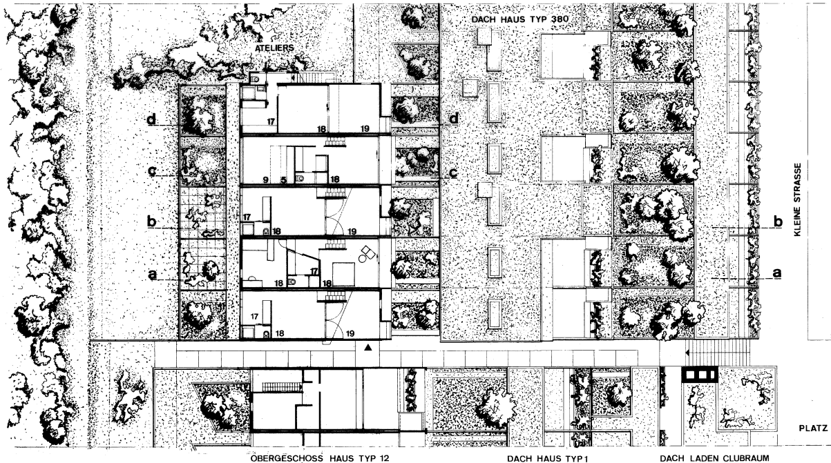
ÜBERGESCHOSS HAUS TYP 12 DACH HAUS TYP 1 DACH LADEN CLUBRAUM HAUS TYP 380 MIT ATELIER, 2.OBERGESCHOSS UND SCHNITTE
