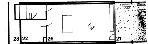
VARIANTEN HAUS TYP 12
